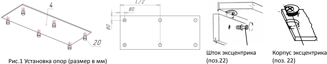
Рис.1 Установка опор (размер в мм) После установки опор произвести их регулировку по месту предполагаемой установки шкафа
