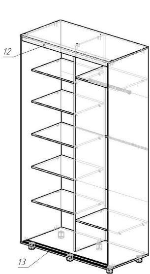
Рис.4 Установка задней стенки
