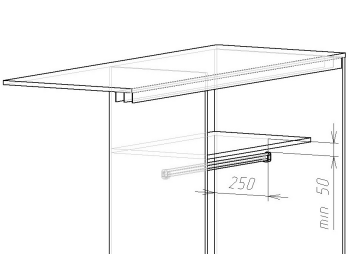
Рис.6 Установка штанги (11) (размер в мм)
