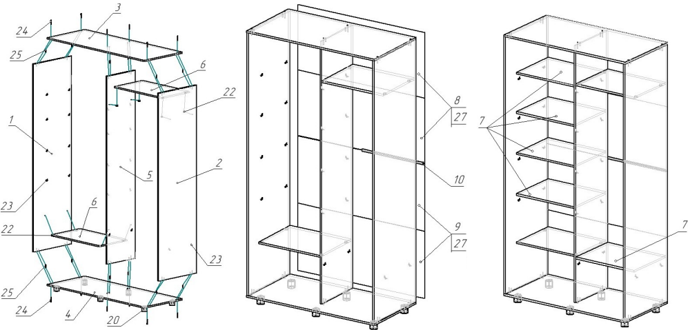
Рис.3 Сборка корпуса
