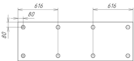
Рис.1 Схема установки опор (размер в мм) После установки опор произвести их регулировку по месту предполагаемой установки шкафа
