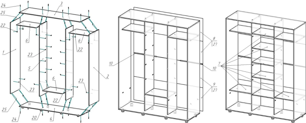
Рис.3 Сборка корпуса
